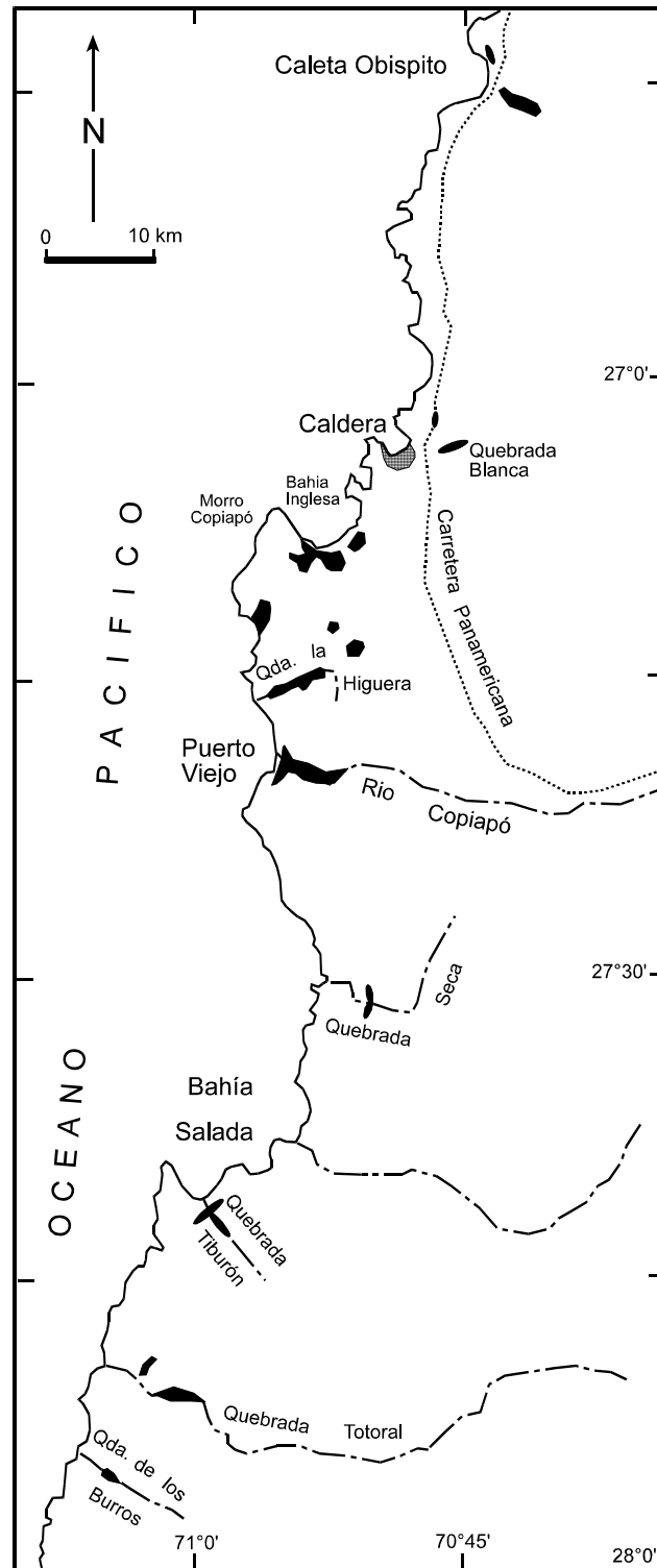
Fig. 1. Área de Estudio y distribución de la Formación Bahía Inglesa, desde Quebrada Obispito (~26°45'S) hasta Quebrada Agua de los Burros (~28°S).
